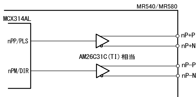
図 2.2-1 ドライブパルス出力信号回路
