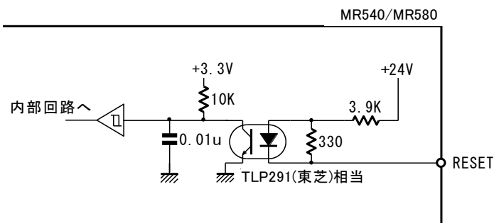
図 2.11-1 リセット入力信号回路
